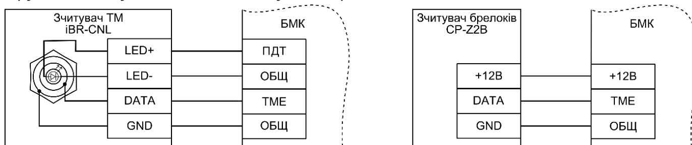
Рисунок 3 - Схема підключення зчитувача ключів TM (зліва) та зчитувача Proximity брелоків (зправа)
