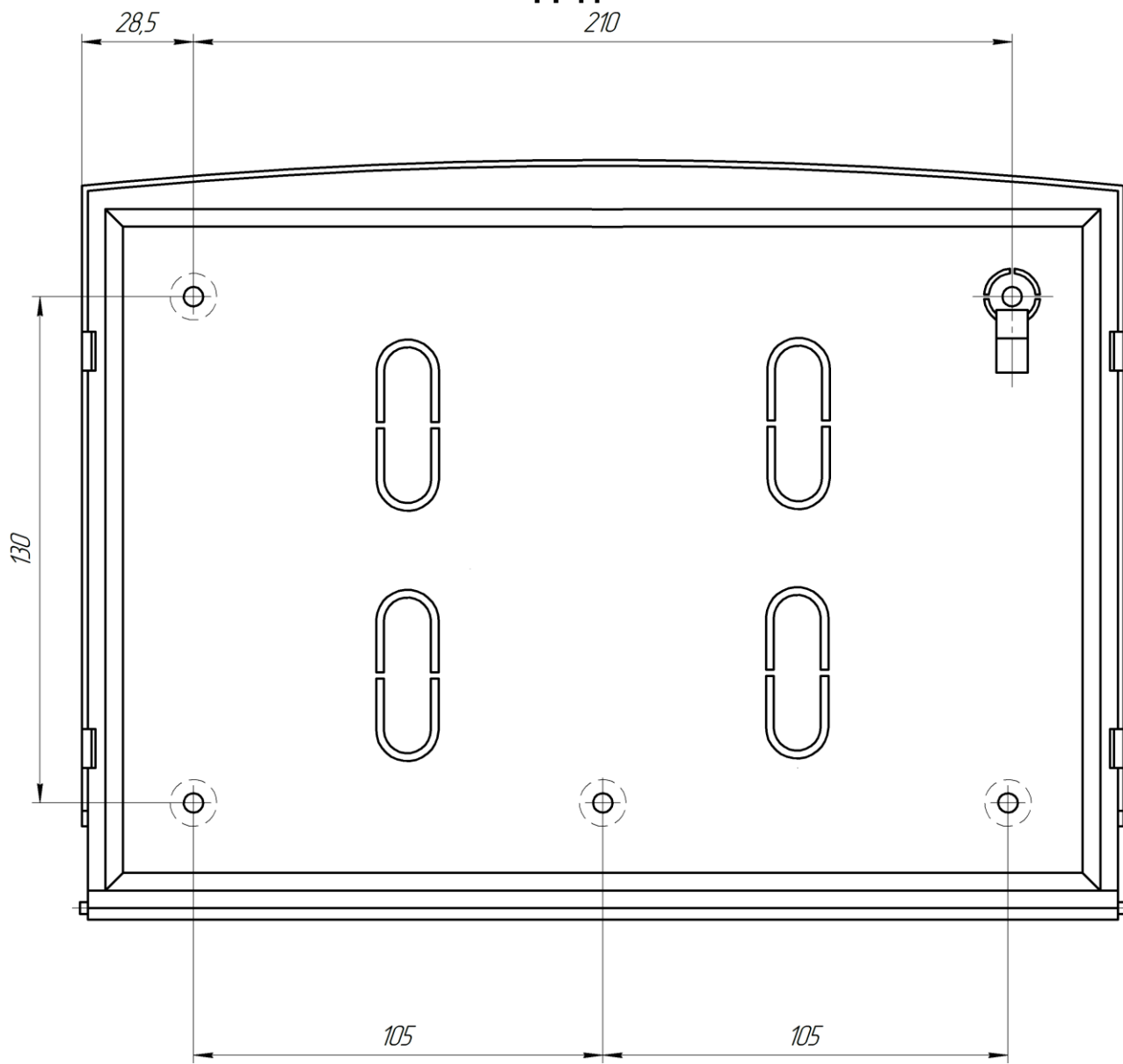
Рисунок В.1 – Установчі розміри ППКО
