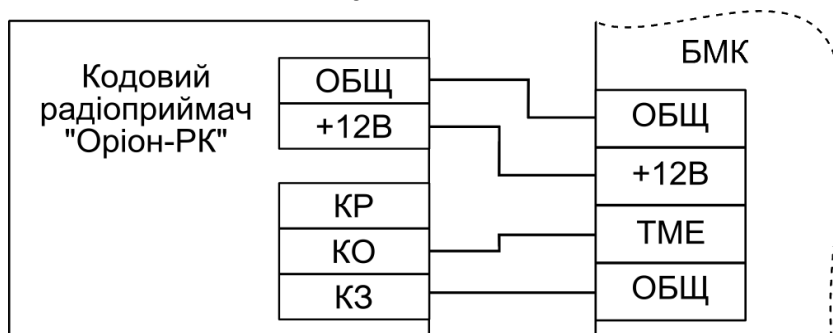
Рисунок 4 - Схема підключення кодового радіоприймача «Оріон-РК»
