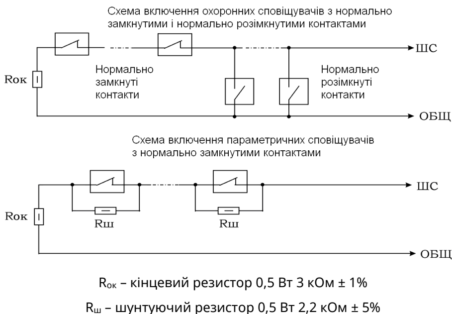
Рисунок 2 – Схеми включення сповіщувачів
