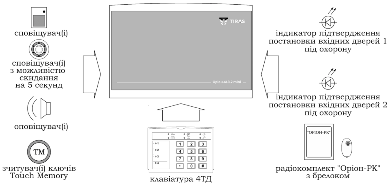
Рисунок 1 – загальний вигляд ППКО «Оріон 4І.3.2 міні»
